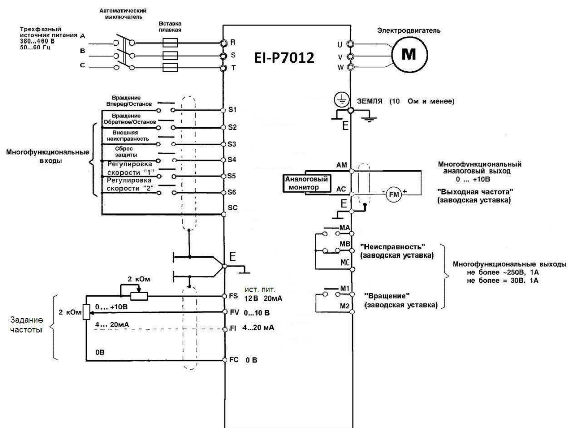
Рис. 9. Схема подключения.
