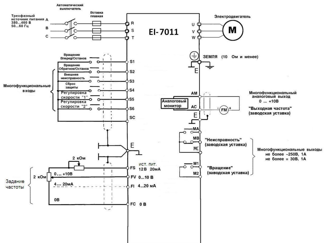
Рис. 9. Схема подсоединения.
