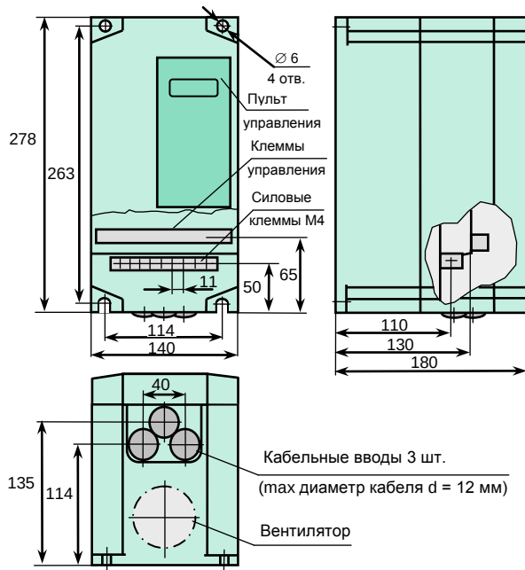
Модели EI-7011 от 001Н до 007Н (от 0,75 кВт до 5,5 кВт)
