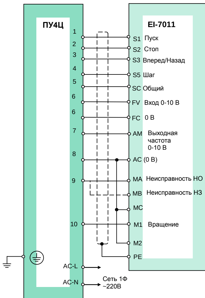
Подключение пульта ПУ4Ц к преобразователю EI-7011
