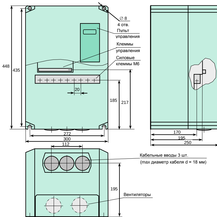
Модели EI-7011 от 020Н до 040Н (от 15 кВт до 30 кВт)
