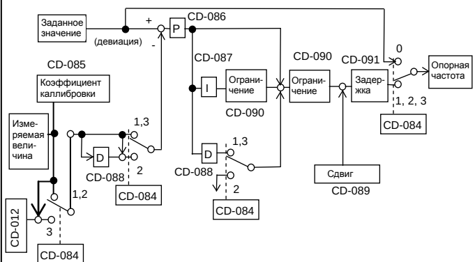
Схема ПИД-регулирования
