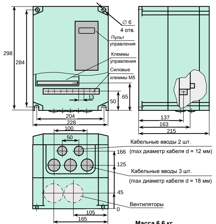
Модели EI-7011 от 010Н до 015Н (от 7,5 кВт до 11 кВт)
