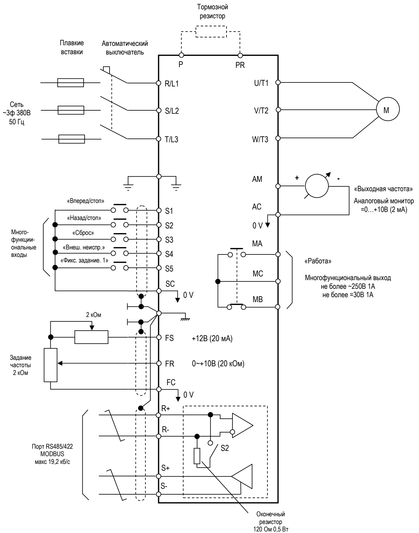
Схема подключения E3-8100
