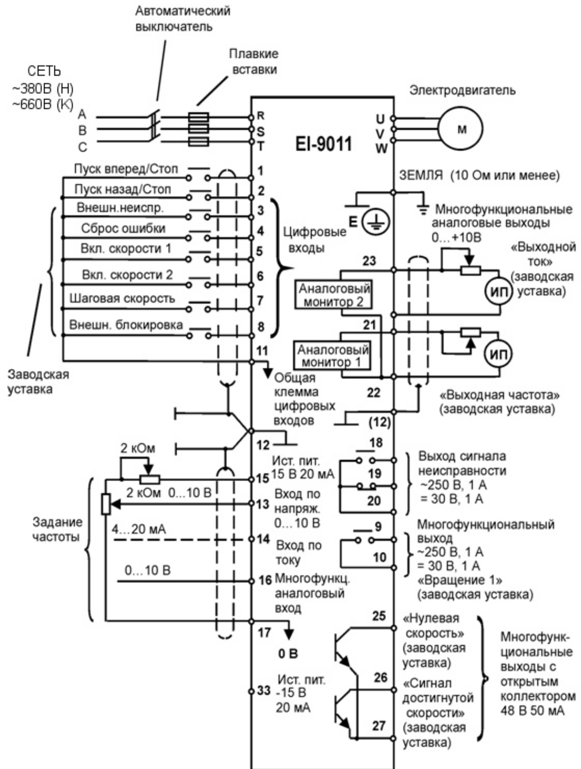
Рис. 4. Схема подсоединения
